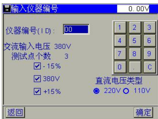
图 4-2-1 稳压精度测量编号设置
