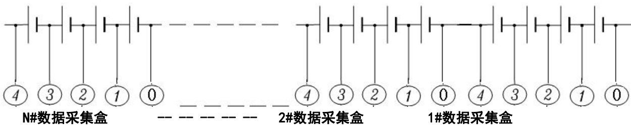
图 3-3-3 多个数据采集盒接线图
