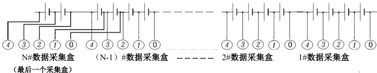
图 3-3-4 电池数量有多余时采集盒接线图
