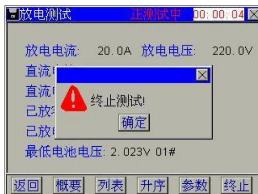
图 4-5-11 电池放电终止测试
